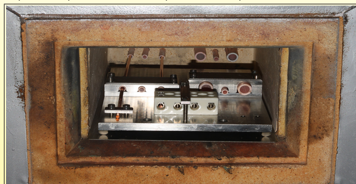
Horno de prueba para determinar la resistividad de la cerámica en función de la temperatura (laboratorio Ultimheat)
